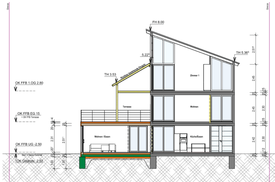
Schnitt S1-1
