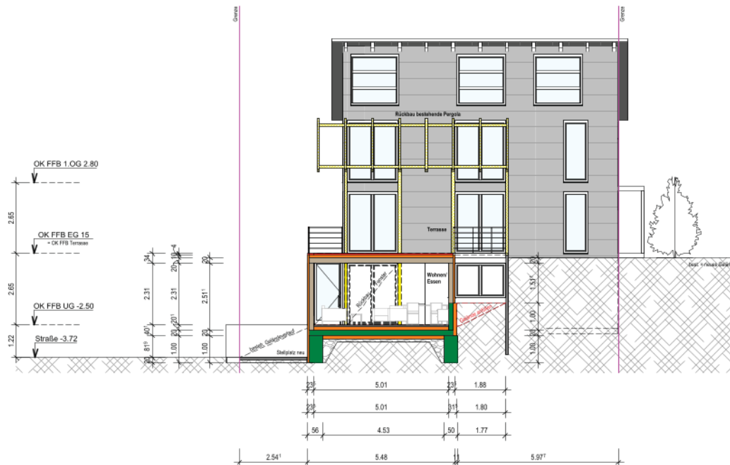
Schnitt S2-2
